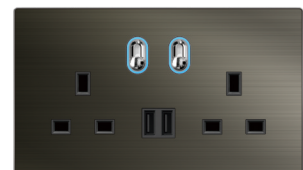
LA-129 146型二位开关带二位13A插座+2USB
